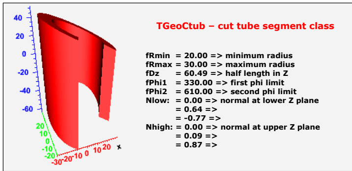
Figure 19-11 TGeoCtub Class
